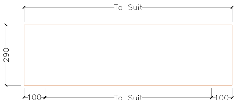
LH5/LH6 - Elevation
